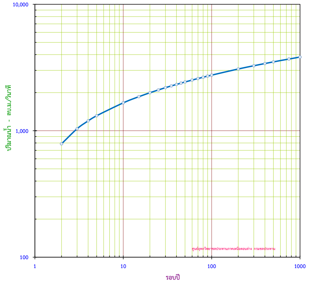
กราฟแสดง ปริมาณน้ำสูงสุดรายปี ขนาดรอบปีต่างๆ สถานี P.2A อ.เมือง จ.ตาก
